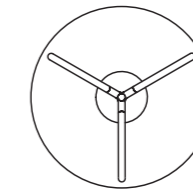
1720 - 1725 Ø: 1200 mm 1720/ H: 720 mm 1725/ H: 440 mm
