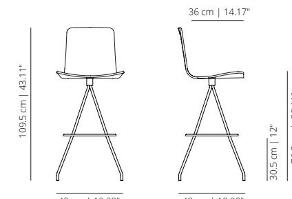
KLTBARTX lacquered
