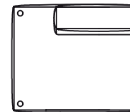
3009-55 open end LHF W1310 x D1070 x H730
