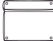
3009-20 2 seater, no-arm W1300 x D1070 x H730
