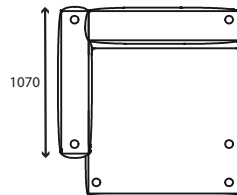
3009-53 mega arm LHF W1300 x D1340 x H730
