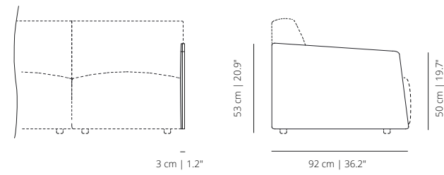
SISBRME medium backrest module
