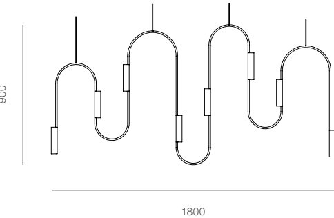
PENDANT E 2 x Module Narrow 3 x Module Link 2 x Module Wide
