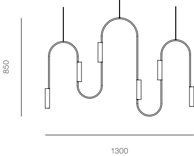
PENDANT D 2 x Module Narrow 2 x Module Link 1 x Module Wide
