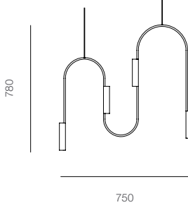
PENDANT C 1 x Module Narrow 1 x Module Link 1 x Module Wide
