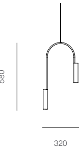
PENDANT A 1 x Module Narrow
