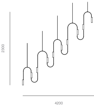
PENDANT I 3 x Module Narrow 4 x Module Link 2 x Module Wide
