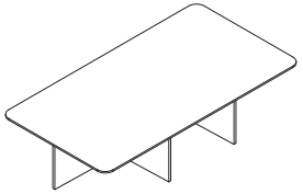
100-2112: glass top 150 100-2111: wood top 150 100-2118: stone top 150 W1500 x D800 x H300
