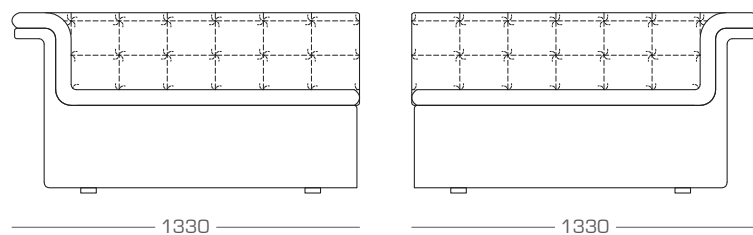
10032-43: 1 arm 133 LHF
