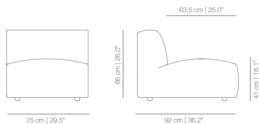
SISB - LOW BACK MODULE
